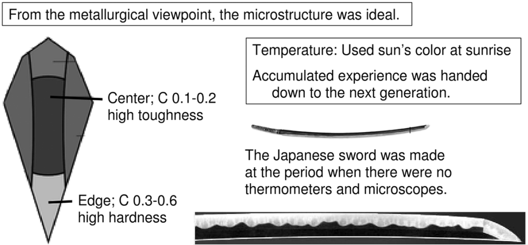
รูปที่ 1 จุดเด่นของดาบซามูไร แหล่งที่มา : Hideo Awaji, 2009 [2]
